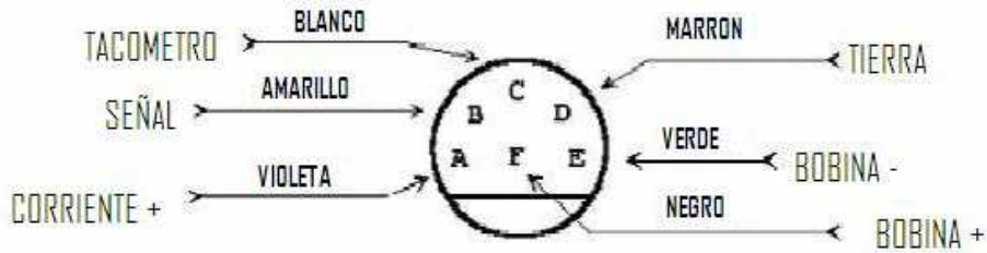
DIAGRAMA DE FICHAS DEL CONECTOR
