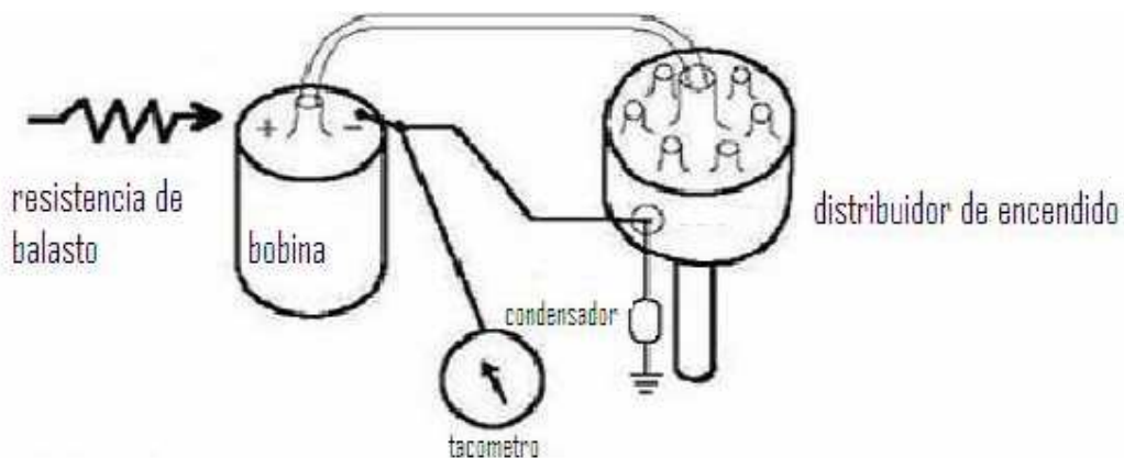
ANTES DE LA INSTALACION DE LA CAJA PERMA-TUNE
